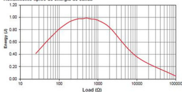
Rendimiento típico de energía de salida
