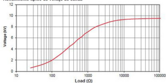
Rendimiento típico de voltaje de salida
